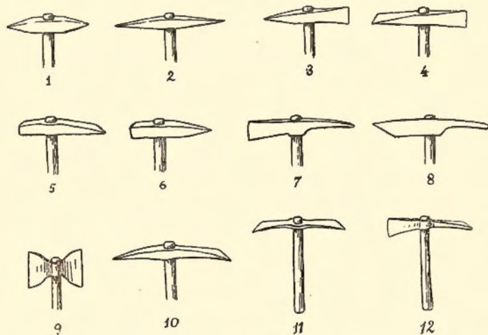
Fig. 2. — 1, pic; 2, escoda, picoleta de dos puntes; 3, puntona, tallant; 4, bec; 5, martell de tall; 6, capmartell, picassó, picot, o martell de punta i testa; 7, xada amb punta; 8, xada amb tall; 9, tallant; 10, puntona; 11, destaló, magall, magalla, magallina, martellina, piccia, picoleta o tallantó; 12, uixol, picotxa o piqueta.
