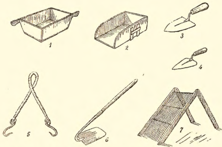
Fig. 1. — 1, gaveta; 2, gavetó; 3, palustre, paleta catalana o esquerrana; 4, paletí; 5, ganxos; 6, lleona o xapo; 7, saranda o porgador.
